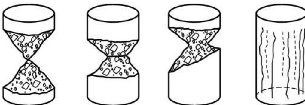
شکل ۳- گسیختگی مناسب آزمونهای استوانه‌ای
